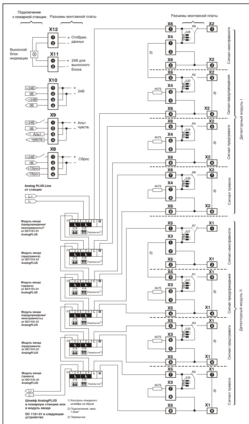
Рис. 5.15: Подключение с применением технологии AnalogPlus
