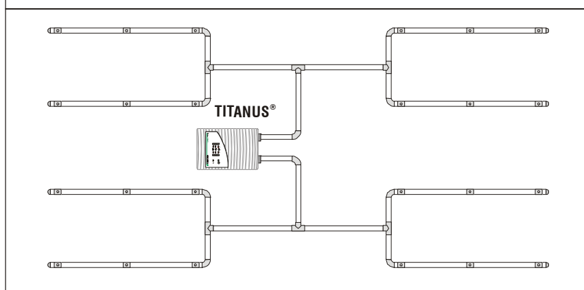
Рис. 4.16: Двойная U-образная система, например, для защиты оборудования
