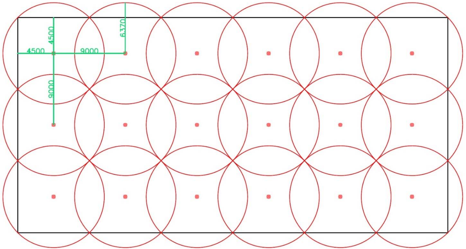
Рис. 3.1, Сетка воздухозаборных отверстий с шагом 9х9м., с учетом радиуса зоны контроля 1 воздухозаборного отверстия равного 6,37м.
