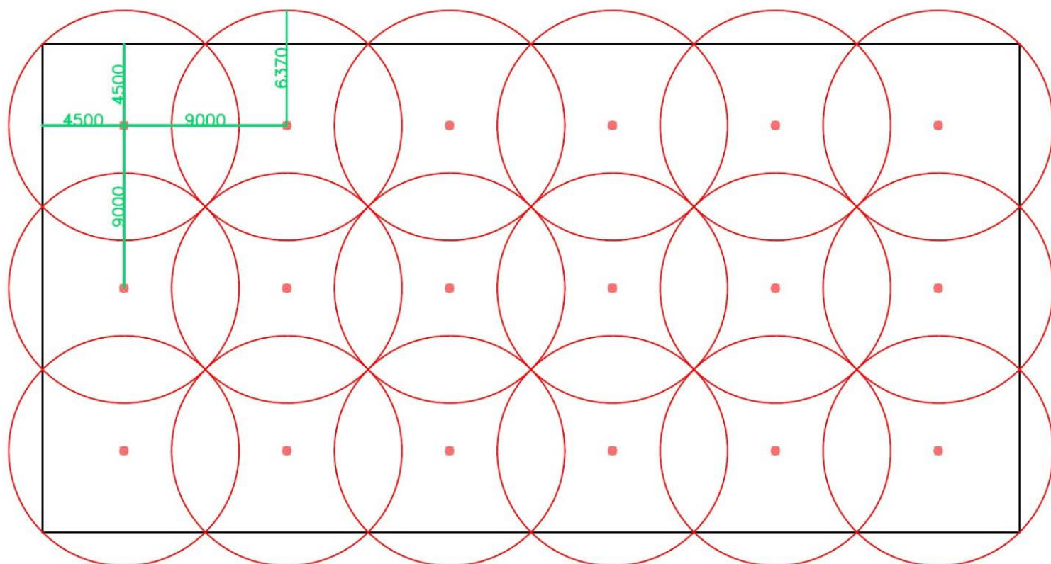
Рис. 3.1, Сетка воздухозаборных отверстий с шагом 9х9м., с учетом радиуса зоны контроля 1 воздухозаборного отверстия равного 6,37м.
