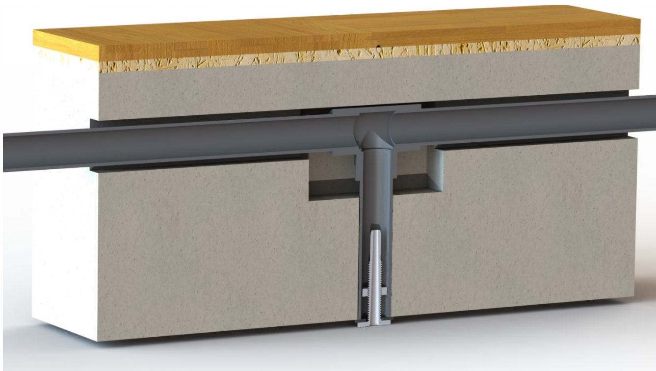
Рис. 4.2.1, Схема размещения аспирационных труб в конструкции здания
