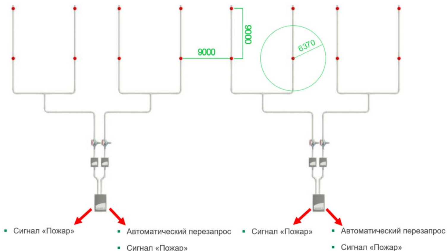
Рис. 5.2.2, Реализация алгоритма В с применением нескольких ИПДА WAGNER TITANUS (Тип TP-1)
