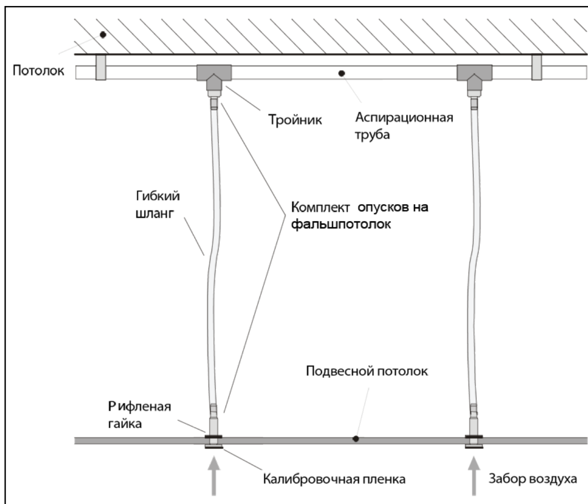
Рис. 4.2.3, Схема размещения аспирационных труб за подвесным потолком
